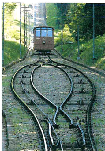
Appareil similaire de type funiculaire
